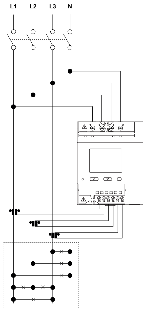
Fig. 3 Trifase con neutro (4 fili).
